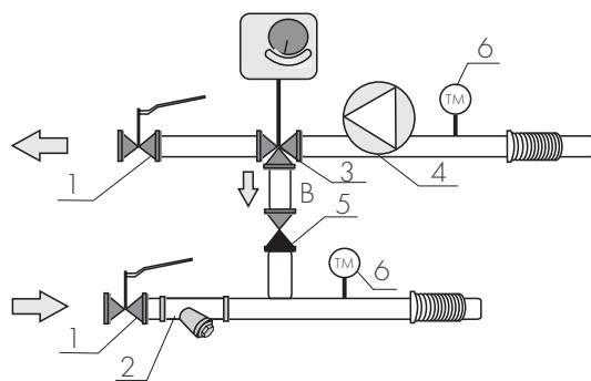
Исполнение 4, с термоманометрами и гибкой подводкой
