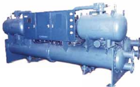
Двухкомпрессорный
