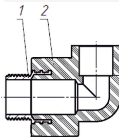
Рисунок 11. Комбинированный фитинг
