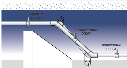
Рисунок 4. Варианты установки компенсаторов
