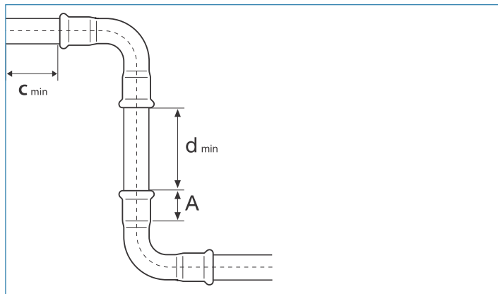
Рис. 60 Монтажные расстояния
