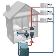
Схема установок JUDO для систем отопления
