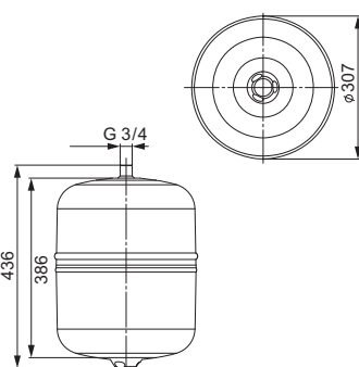
25 литров Расширительный бак
