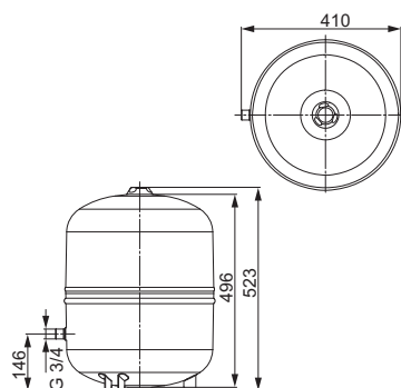
50 литров Расширительный бак
