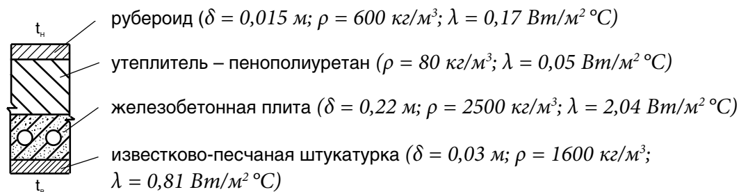
Рис. 7.5. Перекрытие кровли
