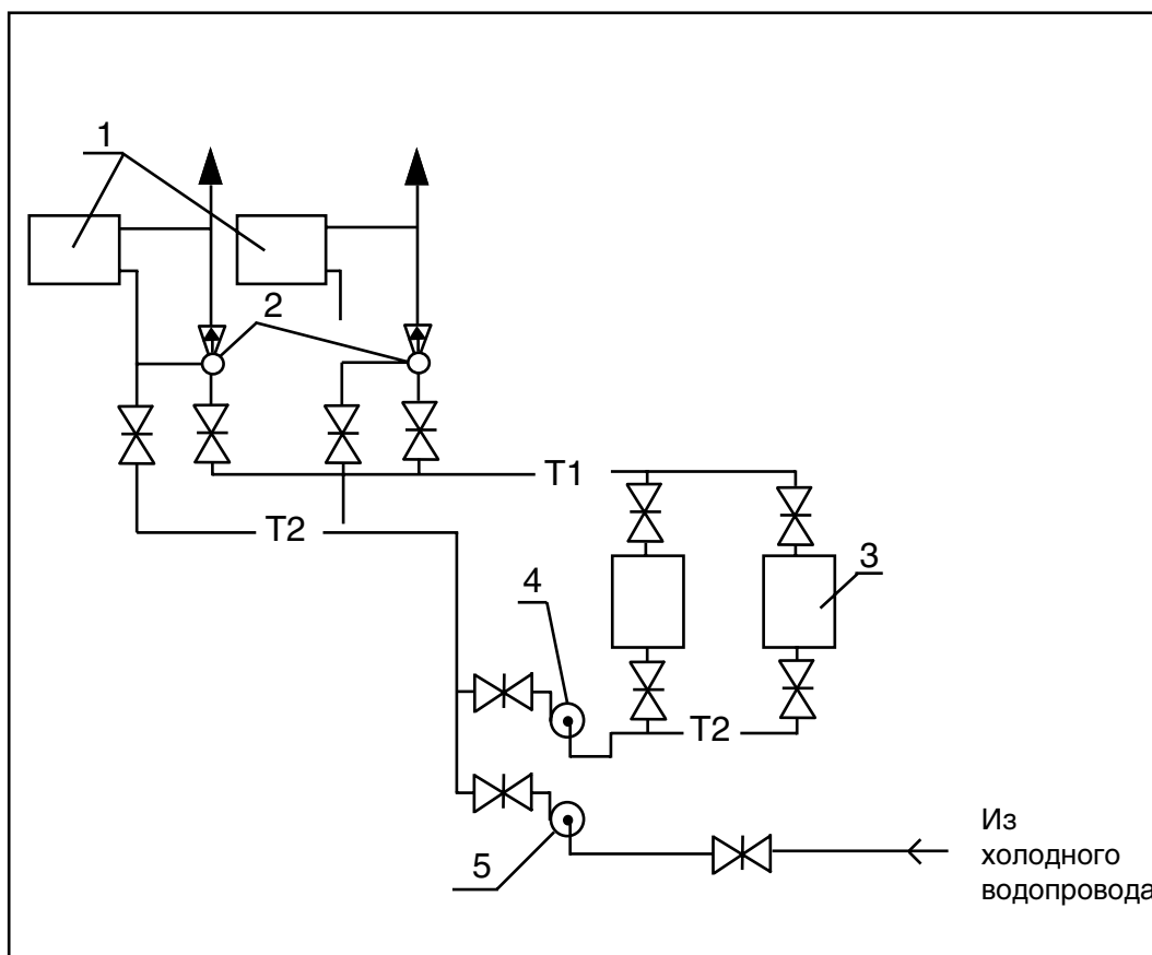
Рис.10.5. Вариант схемы районного водяного отопления. 1. Система отопления; 2. Элеlevator; 3. Котел; 4. Сетевой циркуляционный насос; 5. Подпиточный насос из холодного водопровода.
