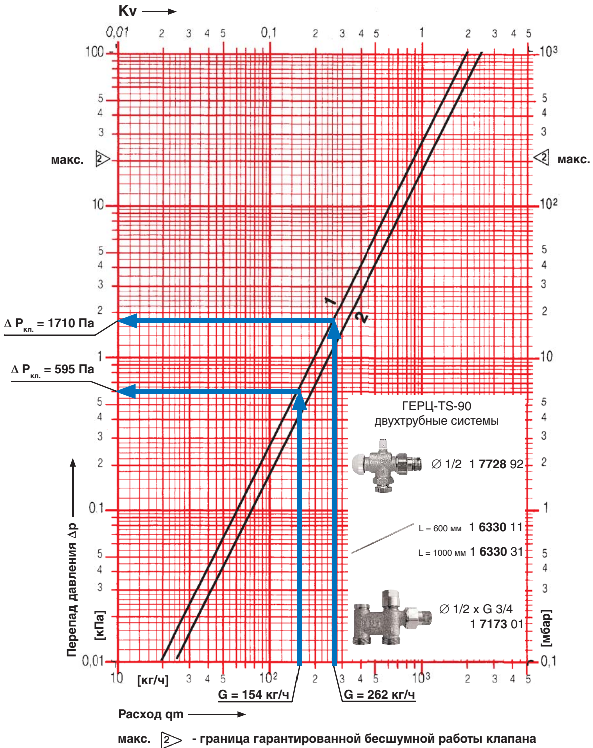
Рис. 7.8.: Пример определения \Delta P_{кв.1} для ветки «А» (262 кг/ч) и для ветки «Е» (154 кг/ч) с помощью номограммы GERЦ-2000, однотрубные системы
