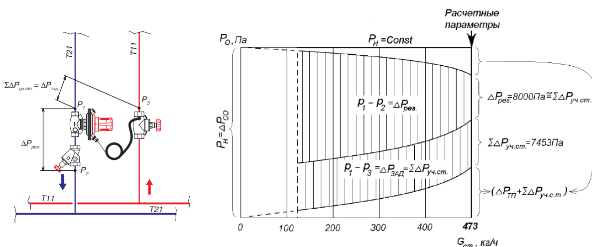
Рис. 6.11.: График изменения перепада давления на регуляторе перепада сителя при использовании циркуляционного насоса с электронным управлением скоростью вращения ротора
