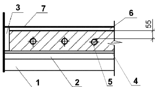
Рис. 9.1.: Конструкция устройства системы подогрева пола
