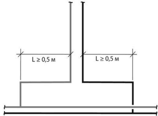
Устройство отступа для компенсации теплового удлинения
