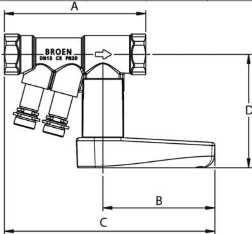
Тип FODRV DN15-50-Присоединение: резьбовое (внутренняя трубная цилиндрическая резьба)
