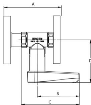
Тип DRV DN15-50-Присоединение: фланцевое
