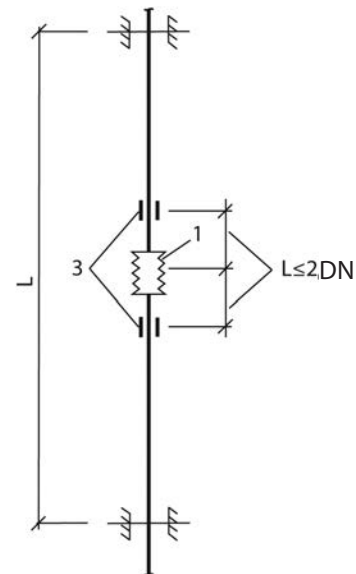
Установка сильфонных компенсаторов
