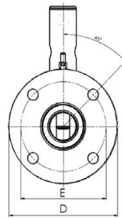
Тип DRV DN65-150 -Присоединение: фланцевое
