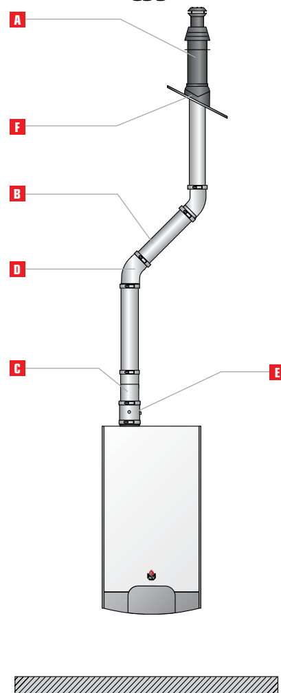
Тип системы дымоотведения S33
