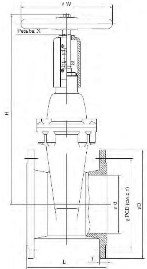
Чертеж габаритный задвижки чугунной с обрезиненным клином пожарной с индикатором положения и неподвижным голым штоком ABRA-A-4010(16)-ixxx
