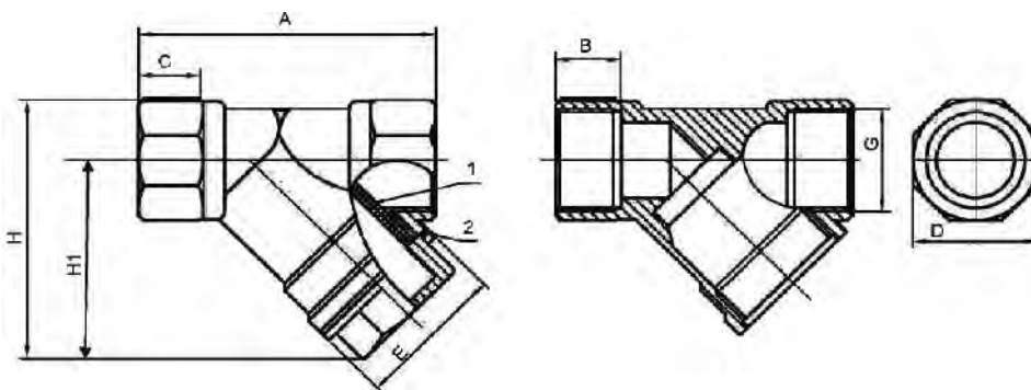
Габаритные размеры, обозначения для заказа, вес и Kv (таблица) фильтра сетчатого латунного резьбового ABRA-YS-3000-E Размеры в мм.
