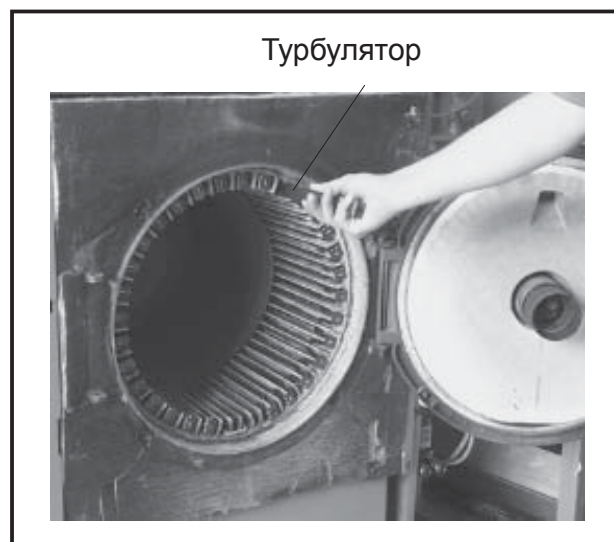
Рис.: Турбуляторы
