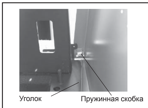
Рис.: Монтаж боковой обшивки
