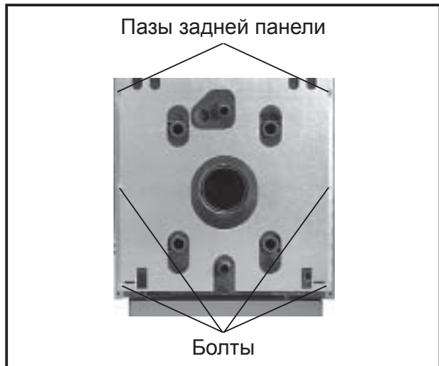
Рис.: Монтаж задней панели
