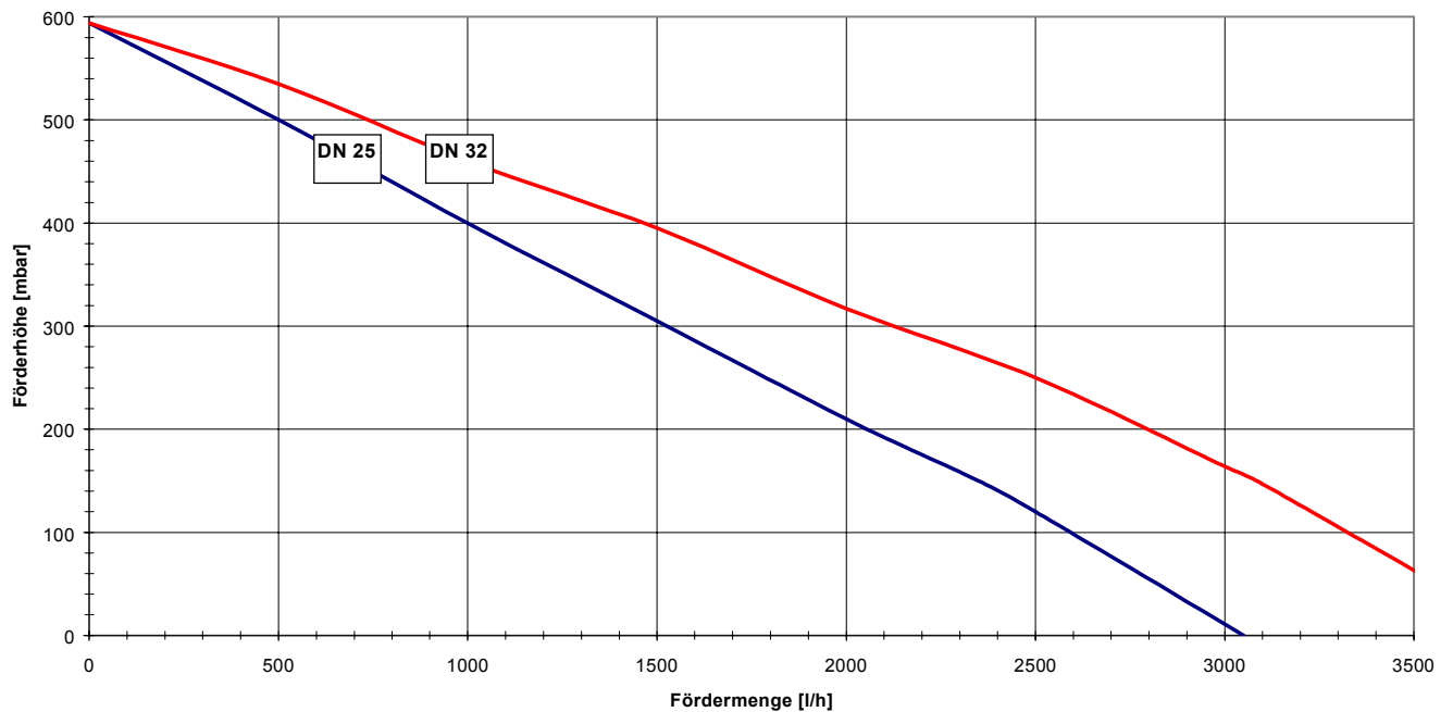
Restförderhöhe Verrohrungsgruppe Heizkreis DN 25 und DN 32
