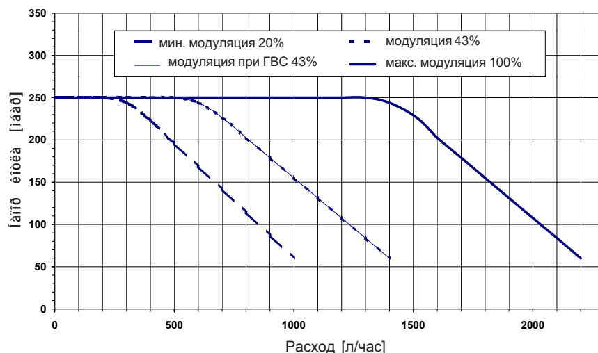
CGB-35 диаграмма насоса с плавной регулировкой числа оборотов
