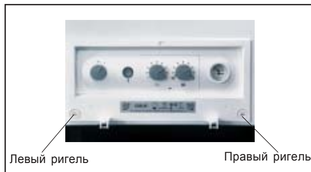
Рис.: Открыть поворотные ригели
