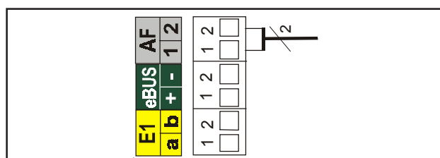
Рис.: Подключение датчика наружной температуры
