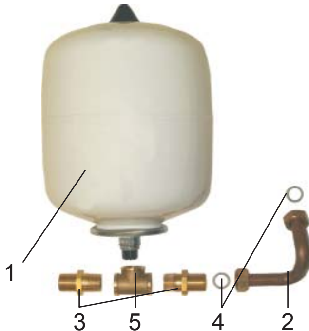
Расширительный бак CS
