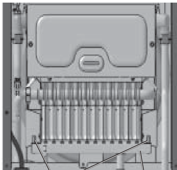
Крепежные винты Газовый штуцер Газораспределительные балки
