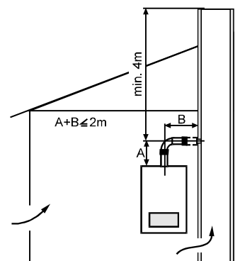
Подключение к дымовой трубе В32 (см. стр. 16)
