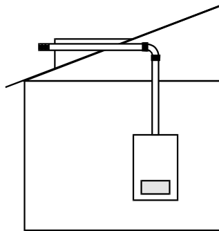
Горизонтальная дымовая труба (с воздуховодом и дымоходом "труба в трубе") ввод через наклонную кровлю С32х (см. стр. 16)
