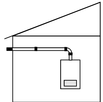
Горизонтальная дымовая труба (с воздуховодом и дымоходом "труба в трубе") ввод через наружную стену С12х (см. стр. 16)
