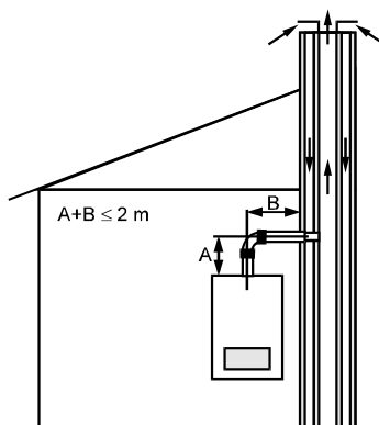
Подключение к дымовой трубе с воздухоподающ. / дымоотв. каналом С42х (см. стр. 16)
