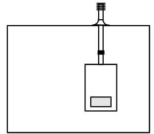
Вертикальная дымовая труба (с воздуховодом и дымоходом "труба в трубе") ввод через плоскую кровлю С32х (см. стр. 15)
