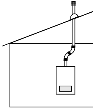
Вертикальная дымовая труба (с воздуховодом и дымоходом "труба в трубе") ввод через наклонную кровлю С32х (см. стр. 15)
