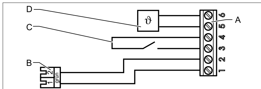
Рис. 4.6 Расположение блока клемм настенного цоколя
