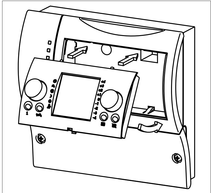
Рис. 4.10 Установка модуля управления ВМ в модуль расширения
