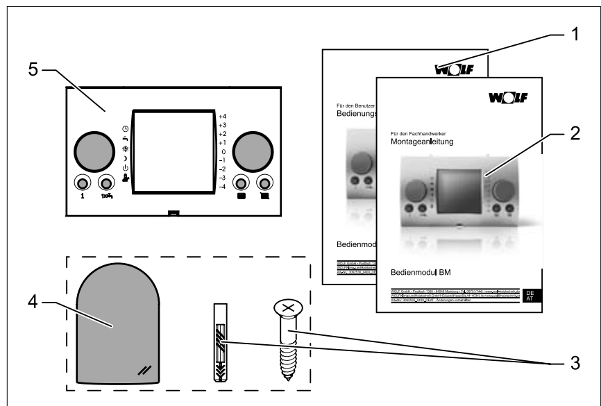
Рис. 4.1 Объем поставки модуля управления ВМ с датчиком наружной температуры/без датчика
