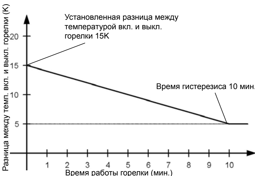
Рис.: Временная зависимость гистерезиса переключения горелки при разнице между температурой включения и выключения горелки, определенной пользователем как 15К, и выбранного времени гистерезиса 10 мин. (параметр HG33)
