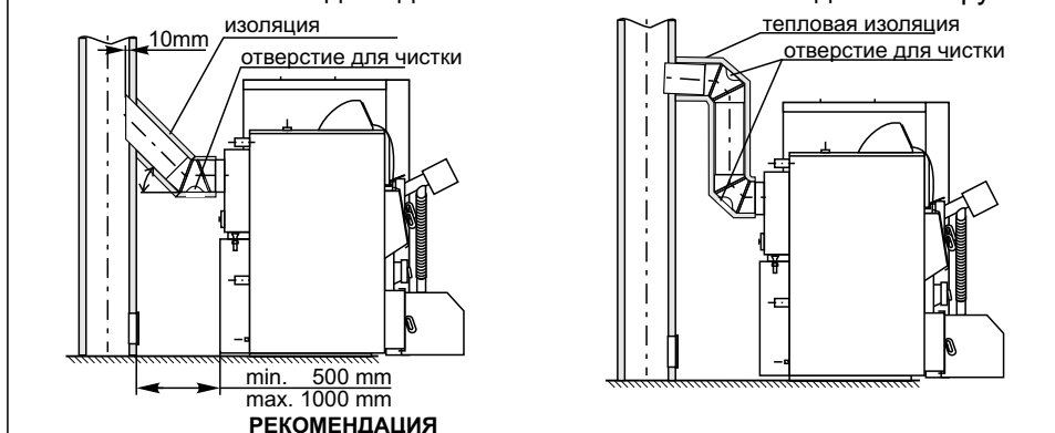
Рис 3. Возможный вид соединения котла ECO-CK Plus к дымовой трубе
