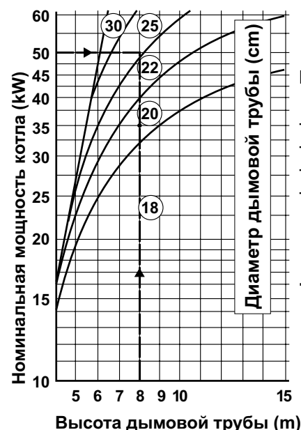
Рис 4. Размеры дымовой трубы для котла ЕКО-СК Plus
