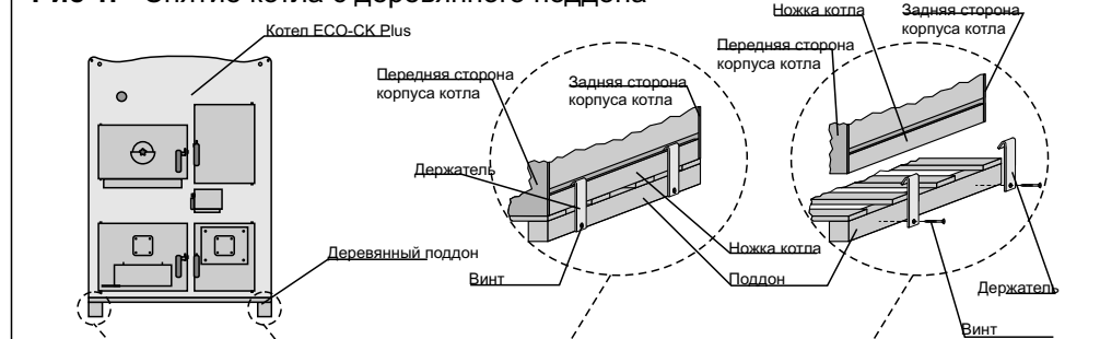
Рис 1. - Снятие котла с деревянного поддона
