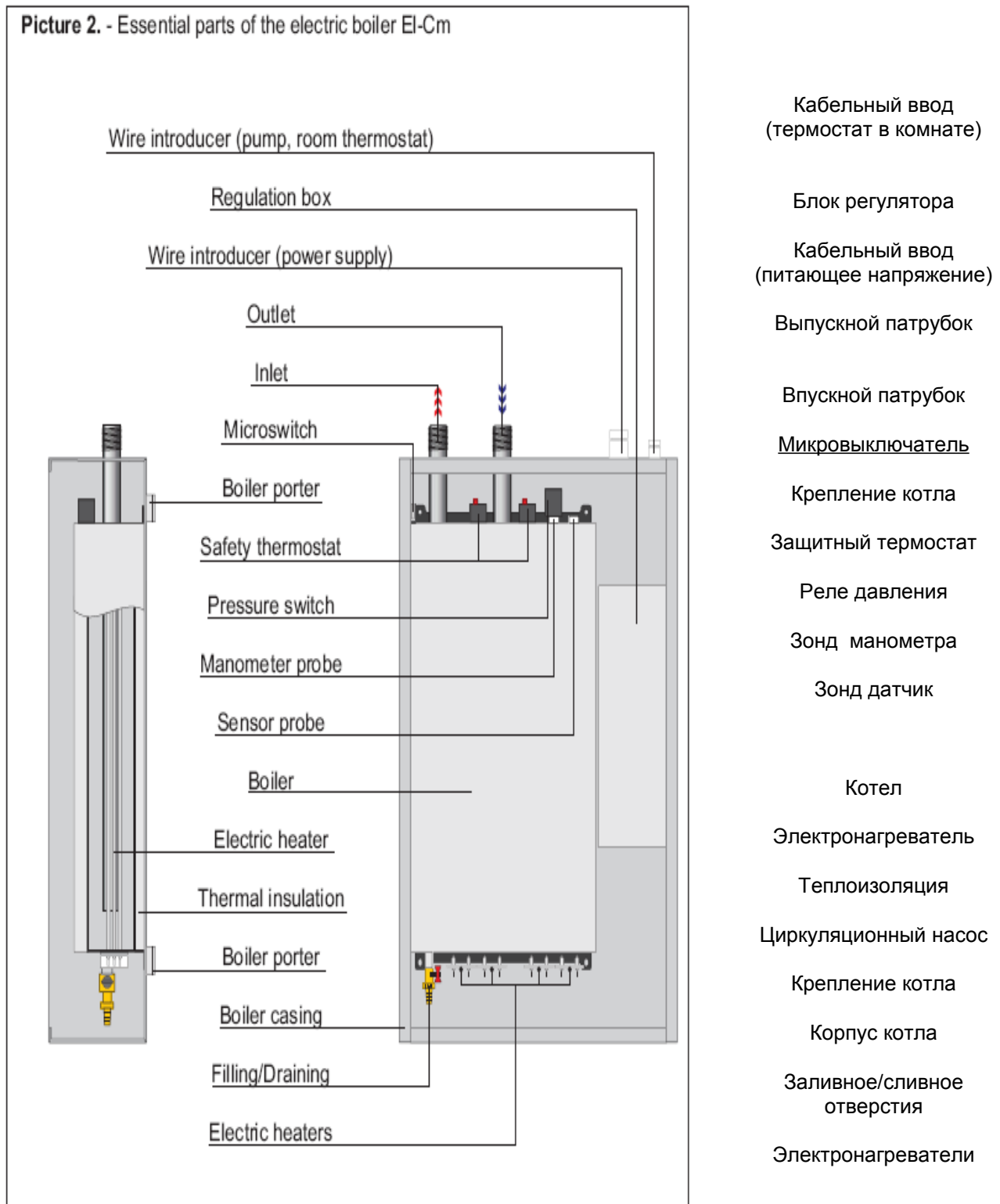
Рис. 2 – Основные компоненты электрического котла EI-Cm Compact
