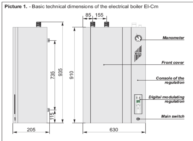
Рис. 1. Основные размеры электрического котла EI-Cm Compact
