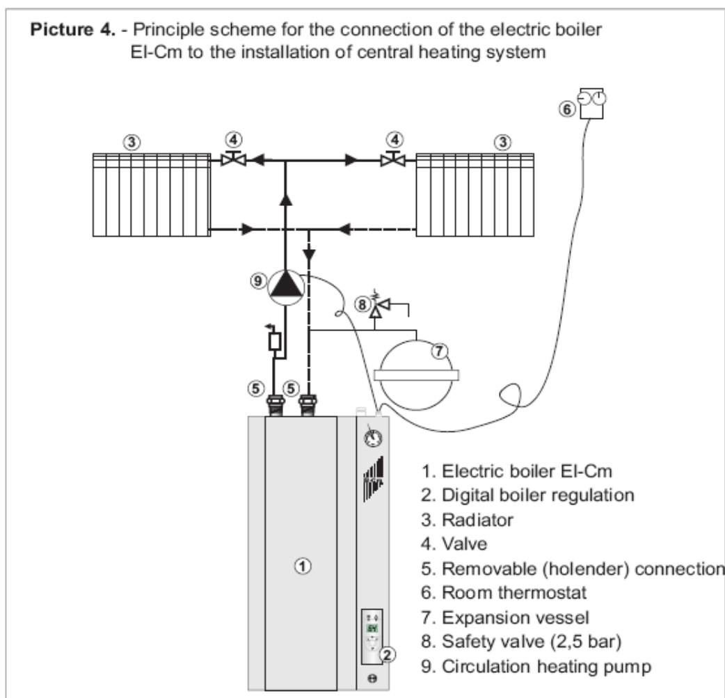
Рис. 4. – Схема подключения электрического котла EI-Cm Compact к системе центрального отопления
