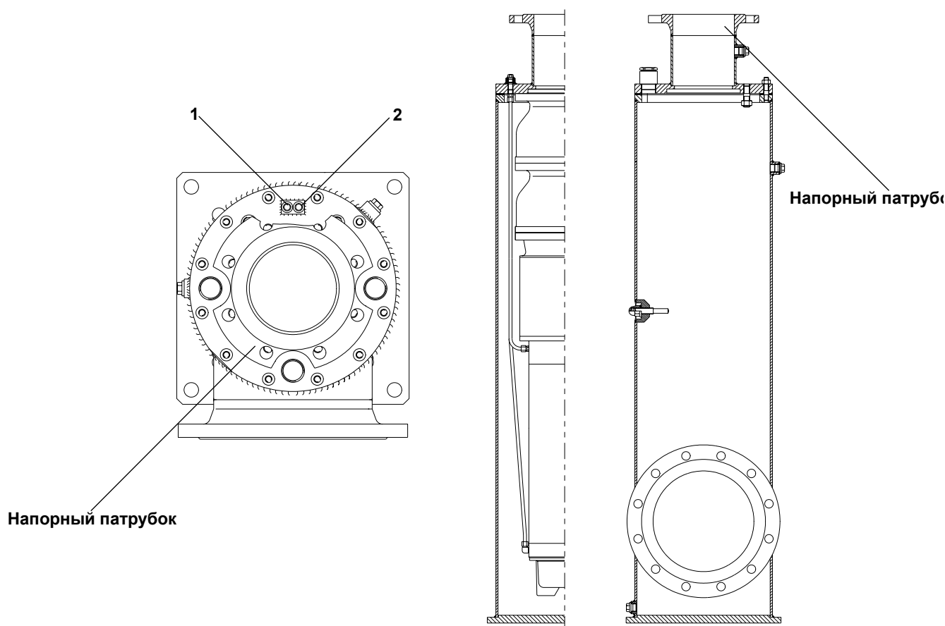
Рис. 5-3: Заполнение двигателя – вертикальный монтаж
