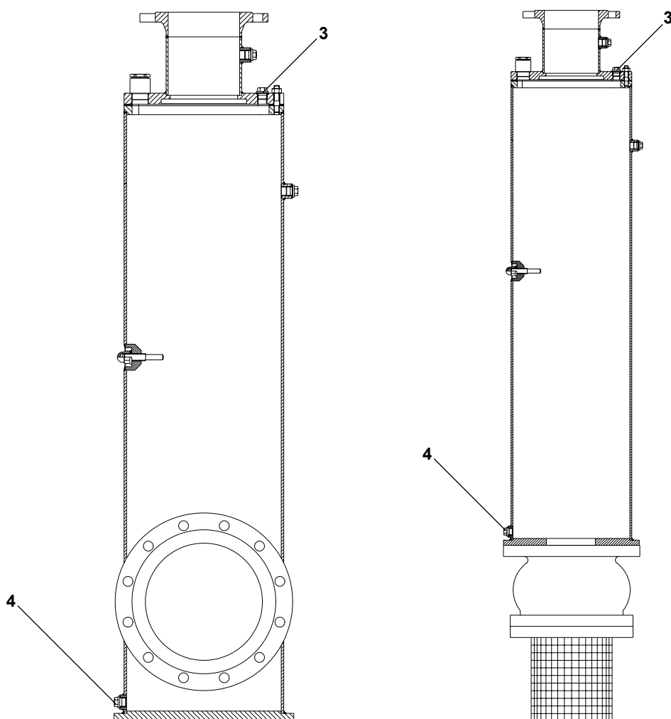
Рис. 5-6: Заливка и опорожнение напорного кожуха при вертикальном монтаже
