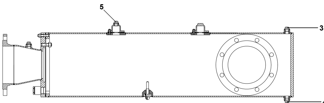
Рис. 5-7: Заливка и опорожнение напорного кожуха при горизонтальном монтаже
