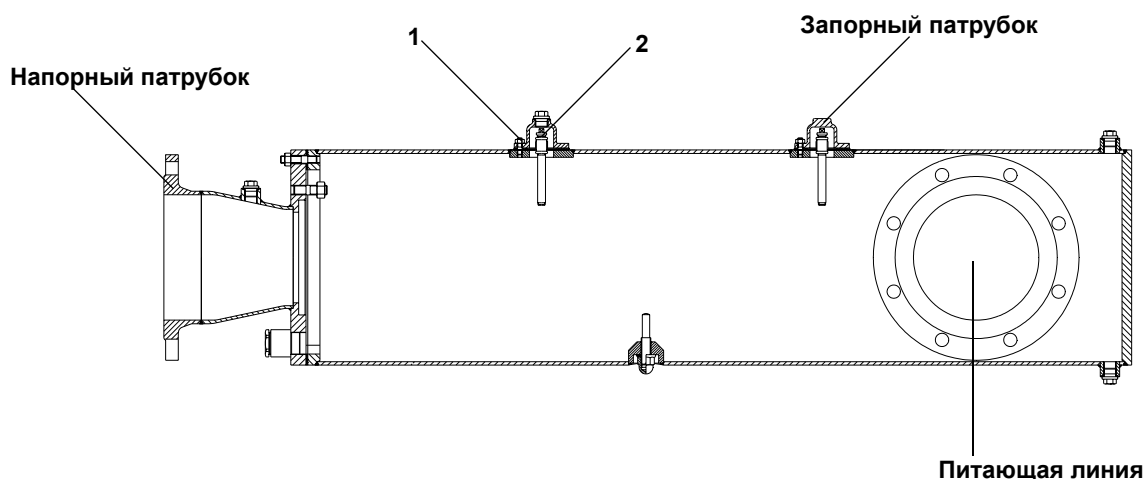
Рис. 5-4: Заполнение двигателя – горизонтальный монтаж
