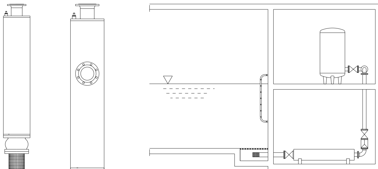
Рис. 5-1: Примеры монтажа
