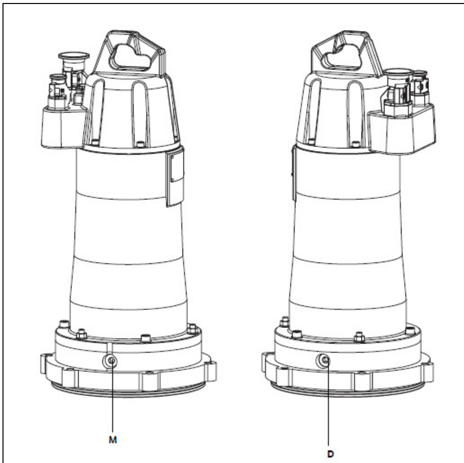
Рис. 7-1: Положение резьбовых пробок
