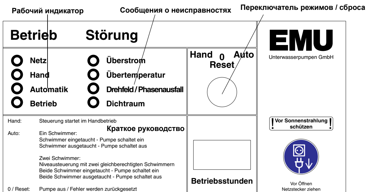
Рис. M-1: Панель управления коммутационного аппарата
