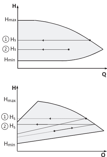
Fig. 42: Регулирование Δp-c/Δp-v
