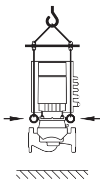
Fig. 7: Транспортировка насоса
