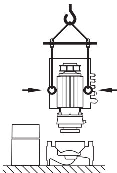
Fig. 23: Транспортировка съемного блока
