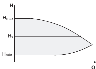
Fig. 14: Регулирование \Delta p-c
