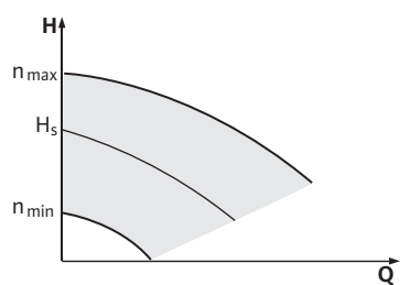
Fig. 43: Ручной режим управления
