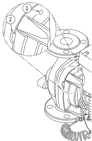
Fig. 46: Резьбовые отверстия и шлицы для отжатия съемного блока от корпуса насоса
