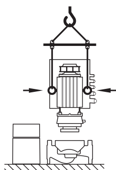
Fig. 8: Транспортировка съемного блока
