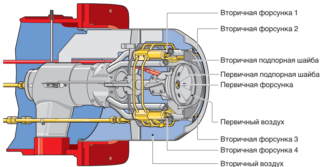
Смесительное устройство
