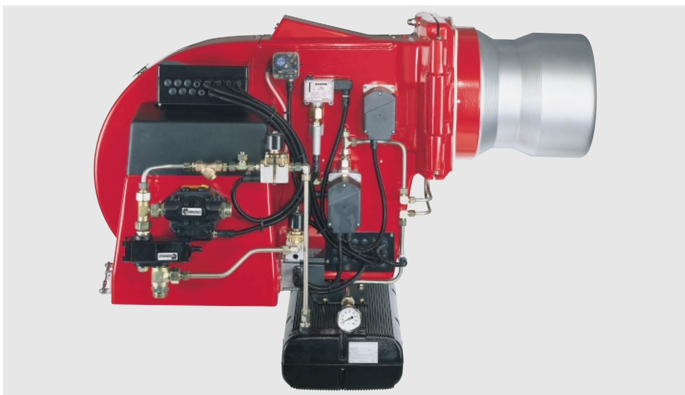
Жидкотопливная горелка Weishaupt RMS50/2-A с цифровым менеджером горения
