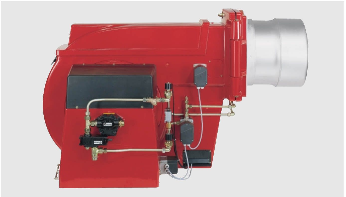
Жидкотопливная горелка Weishaupt RL70/2-A с цифровым менеджером горения
