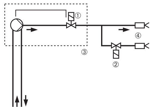
Функциональная схема горелки WL20-2/C, исп. Z
