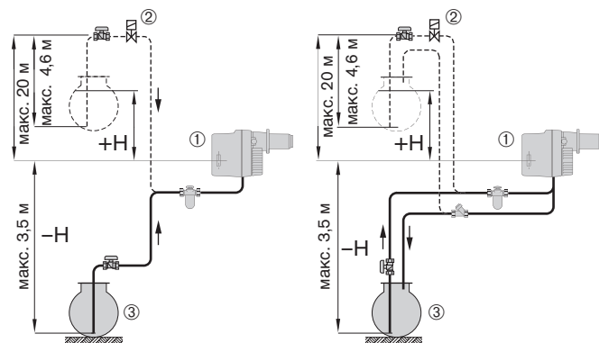
Однотрубная система
