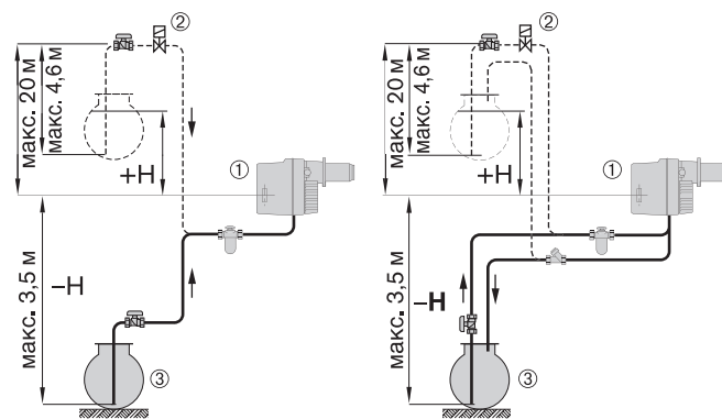
Однотрубная система Двухтрубная система
