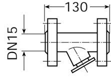
Диаметр DN15
