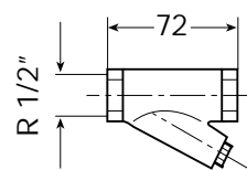
Диаметр R 1/2"
