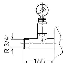
Диаметр R 3/4"
