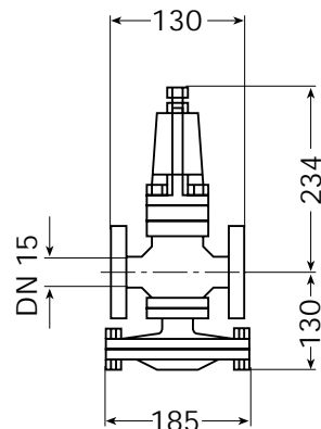
Диаметр DN15
