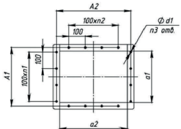
Фланец нагнетания
