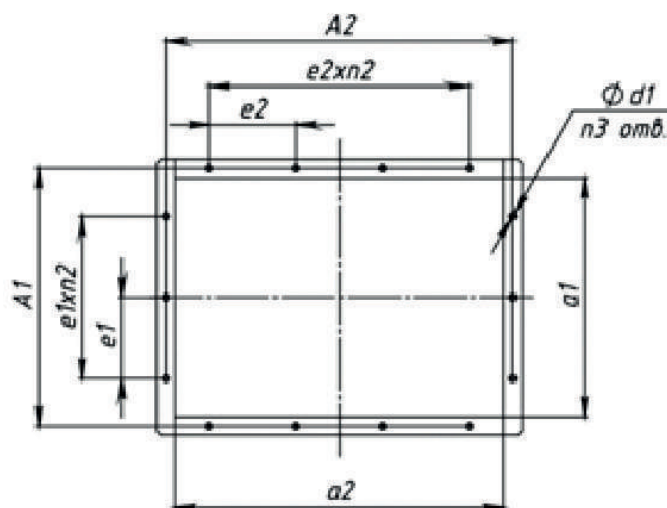
Фланец нагнетания
