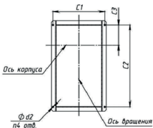
Схема расположения отверстий под фундаментные болты
