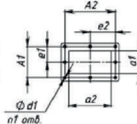
Фланец нагнетания
