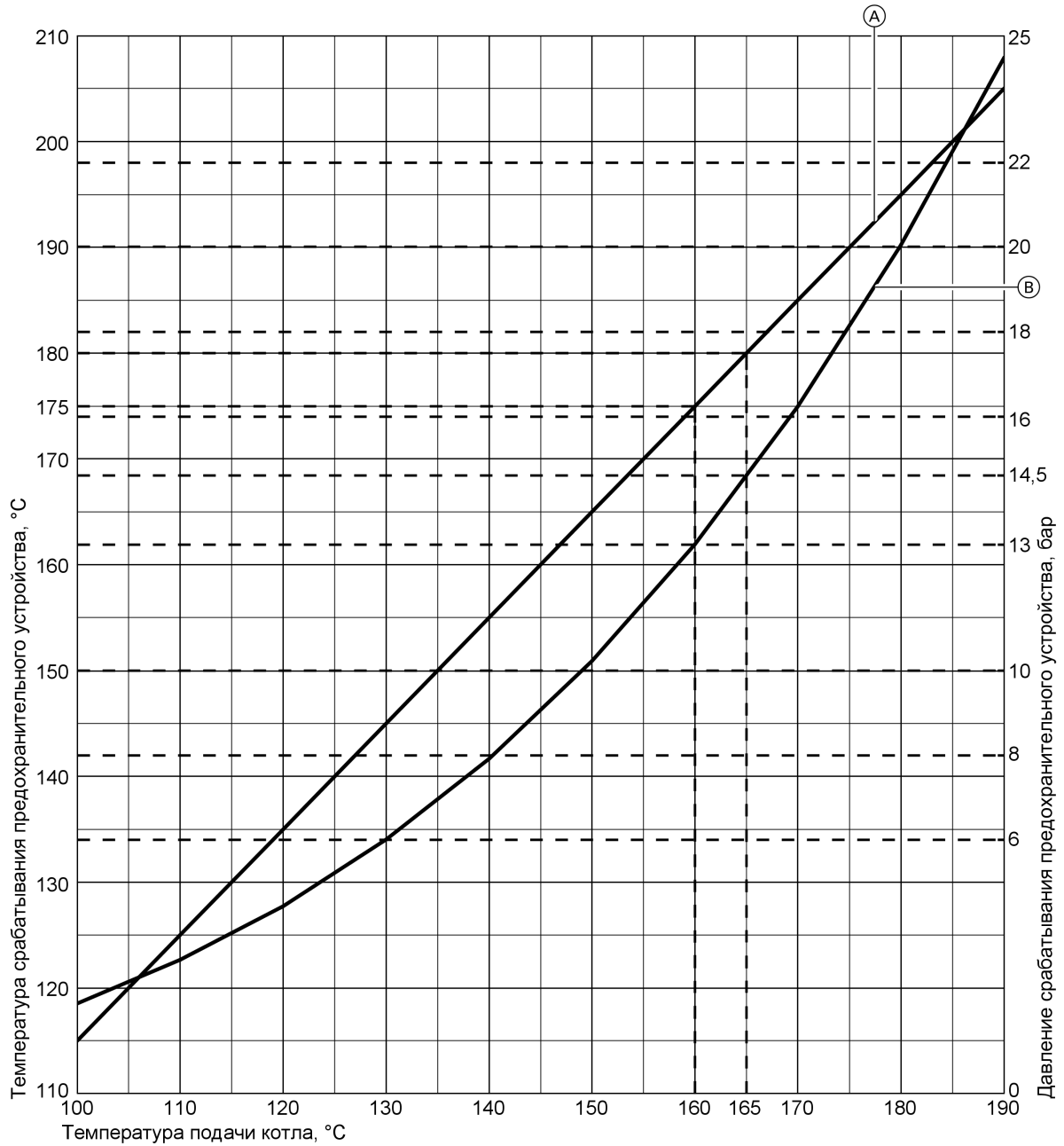
Диаграмма 1. Зависимость температуры и давления срабатывания предохранительного устройства от температуры подачи котла
