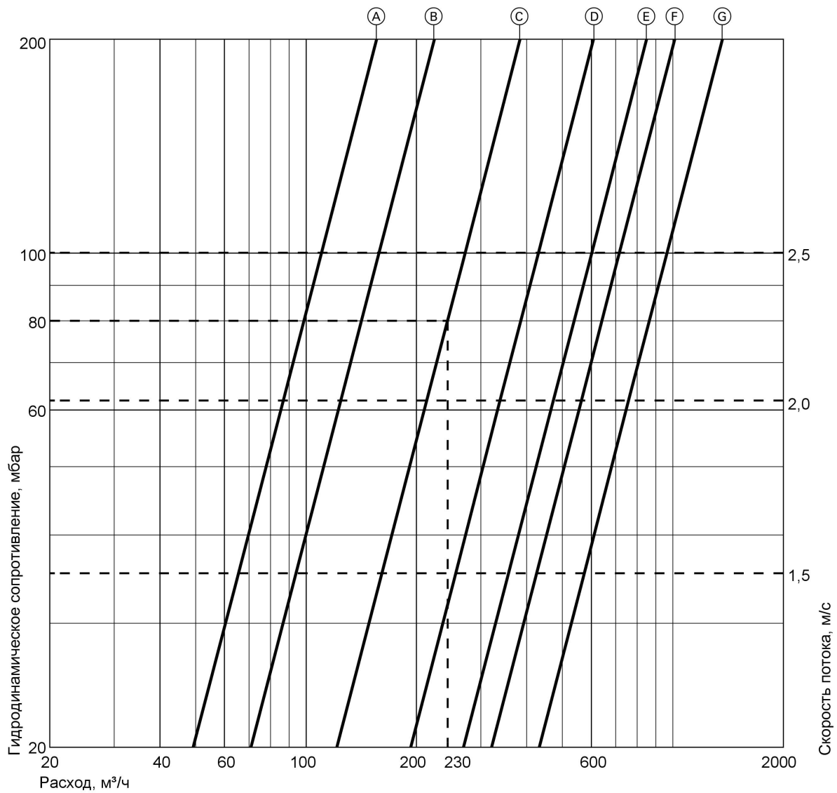
Диаграмма 5. Гидродинамическое сопротивление на стороне греющего контура
