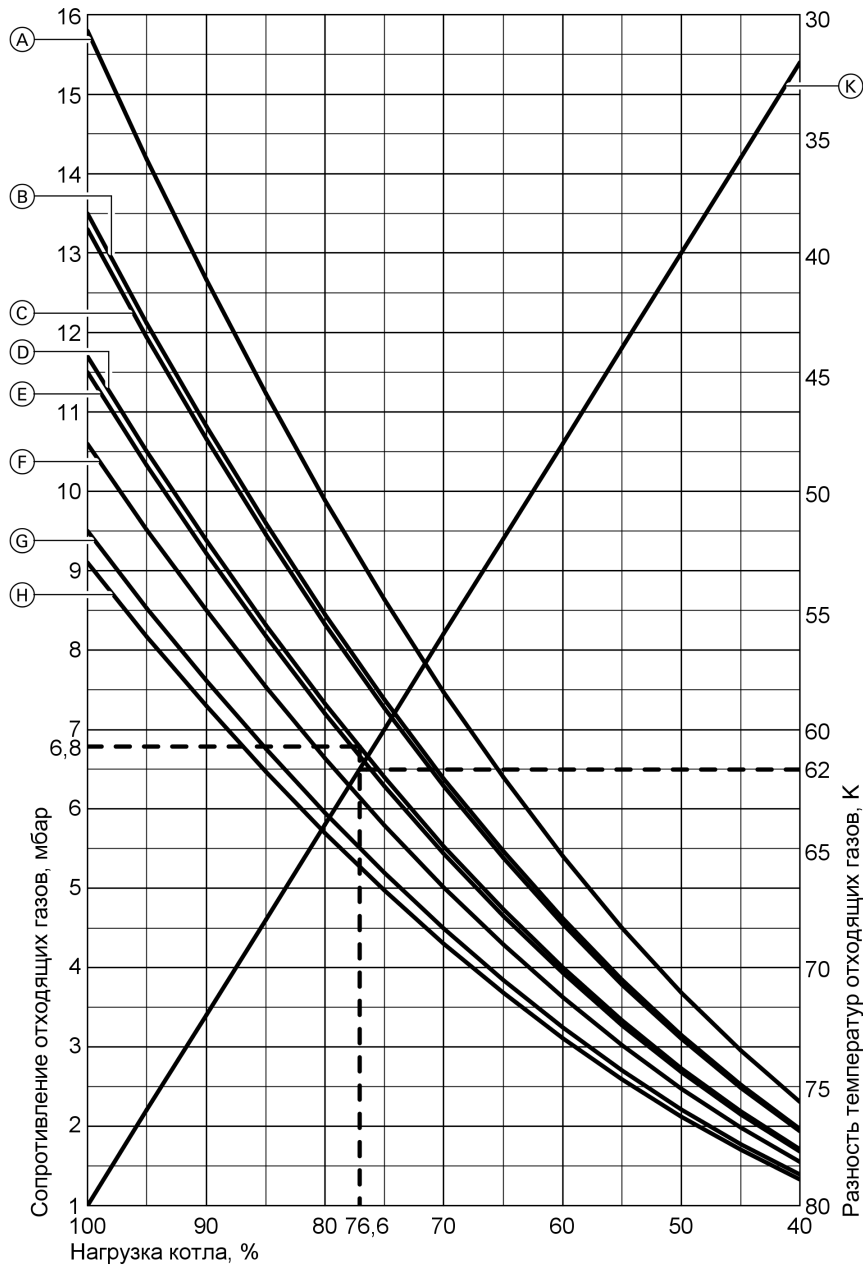
Диаграмма 3. Зависимость сопротивления и разности температур уходящих газов от мощности котла
