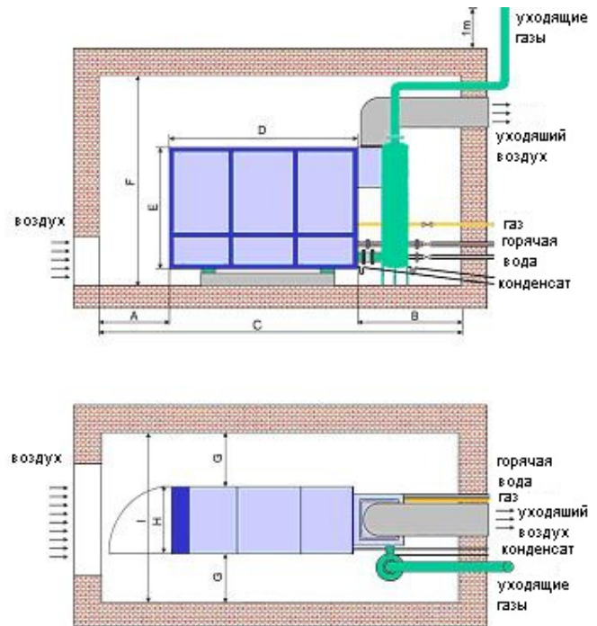
Рис.9 Схема приточно-вытяжной вентиляции в помещении
