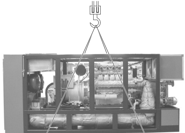
Рис. 4 Транспортировка краном с помощью тросов. Требуются четыре транспортировочных петли
