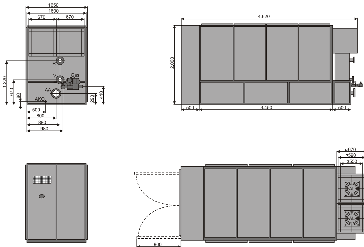
Рис. 1 Габаритные и присоединительные размеры VITOBLOC 200 EM-238/363 (размеры в мм); Установленный короб вентилятора на задней панели можно демонтировать для транспортировки модуля.
