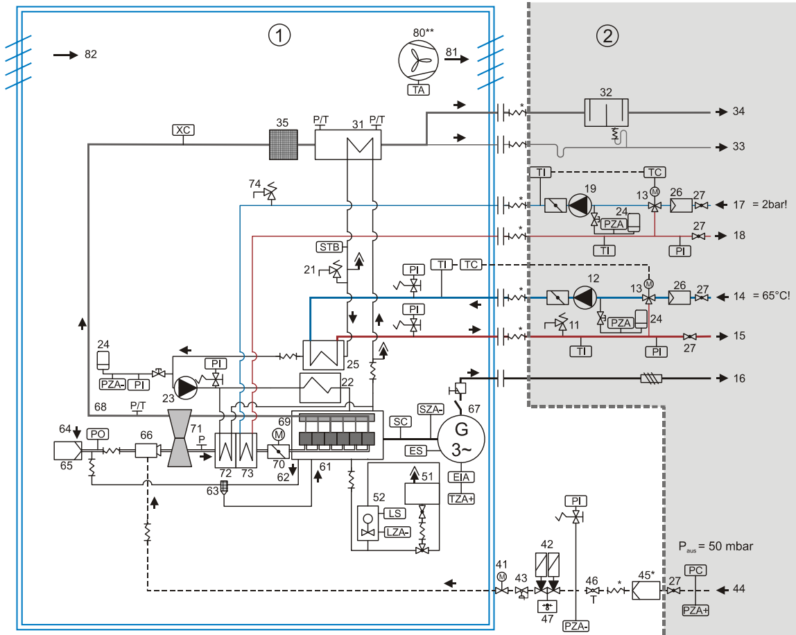
Рис. 2 Контрольные устройства, исполнение Vitobloc 200 EM-401/549 с отдельным низкотемпературным контуром; (поз. 80 и 83 опционально) Если давление системы в контуре охлаждения наддувочного воздуха (17+18) превышает 2 бар, то заказчик должен предусмотреть гидравлический разделитель!
