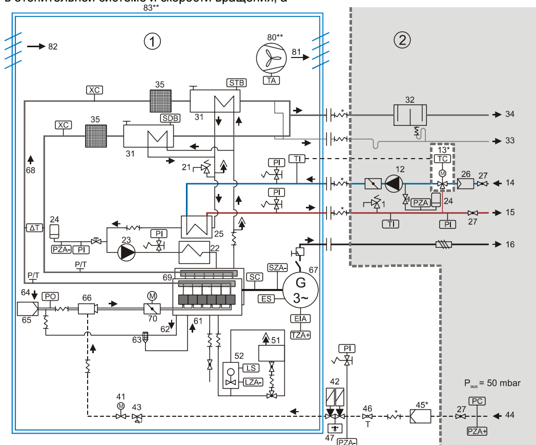
Рис. 2 Устройства контроля
