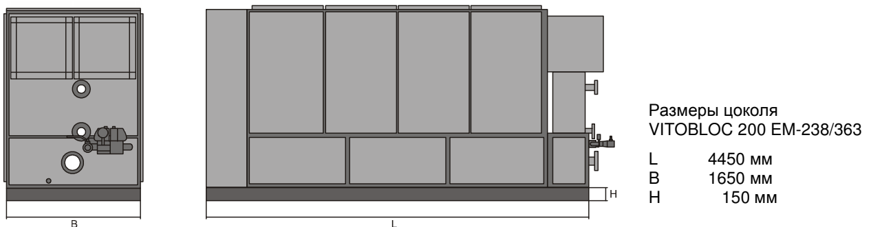
Рис. 7 Размер цоколя
