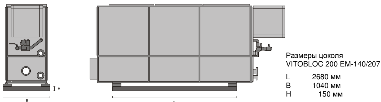
Рис.7 Размер цоколя
