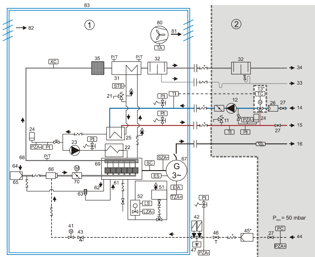
Рис.2 Устройства контроля
