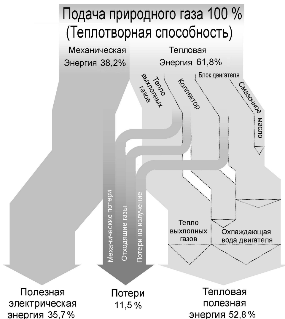
Рис. 1 Энергетический баланс модуля
