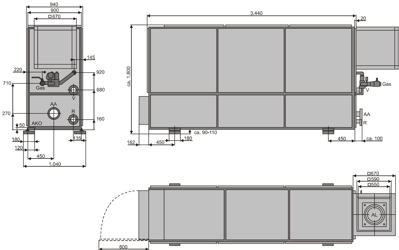
Рис.5 Размеры и подключения VITOBLOC 200 EM-140/207 (размеры в мм); Установленный короб вентилятора на задней панели можно демонтировать для транспортировки
