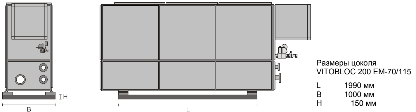
Рис. 7 Размер цоколя
