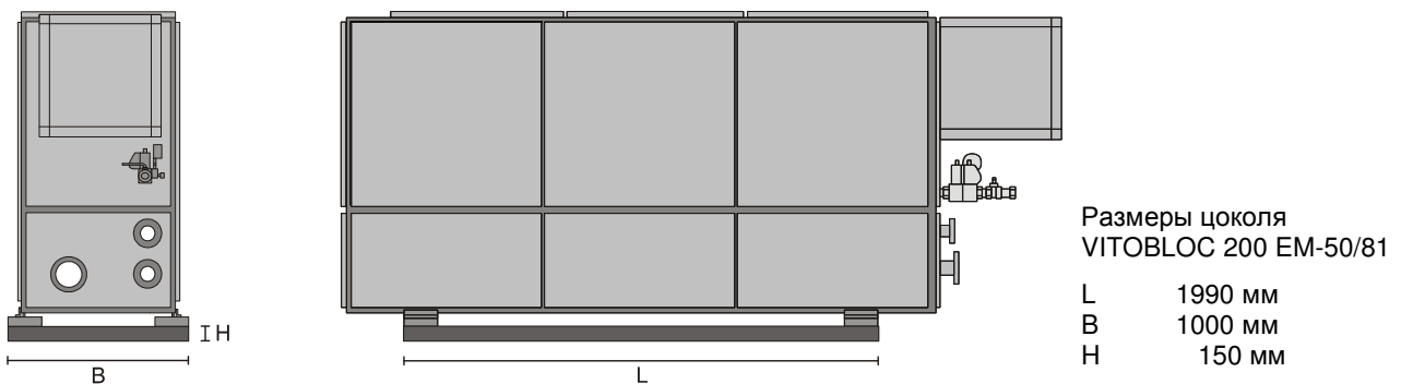
Рис. 7 Размер цоколя
