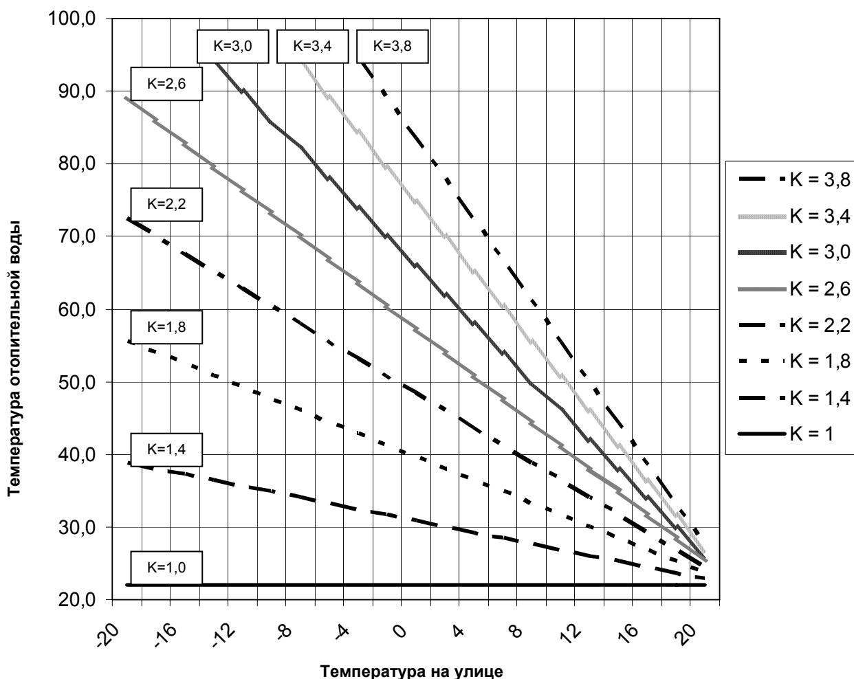
Зависимость температуры отопительной воды от температуры на улице, Требуемая температура в помещении 22 °C
