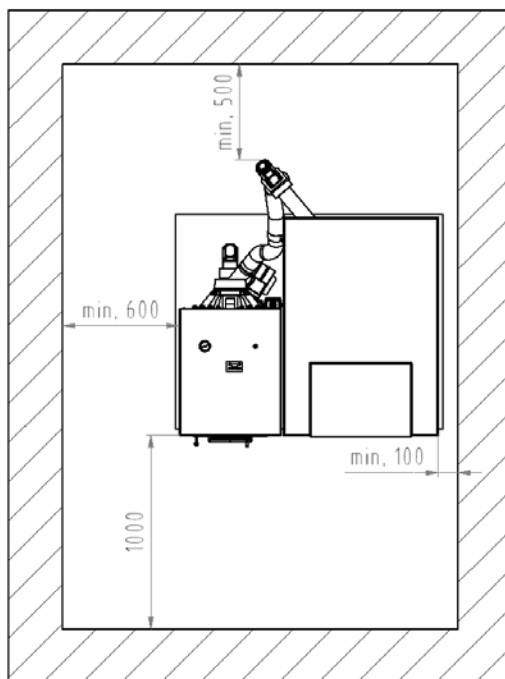
Рис. 6 Расположение котла VIADRUS HERCULES ECO в котельной
