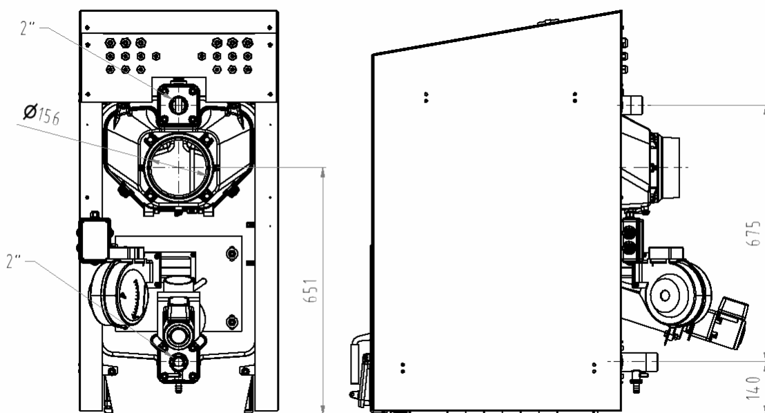
Рис. но. 8 Присоединительные размеры котла VIADRUS HERCULES ECO
