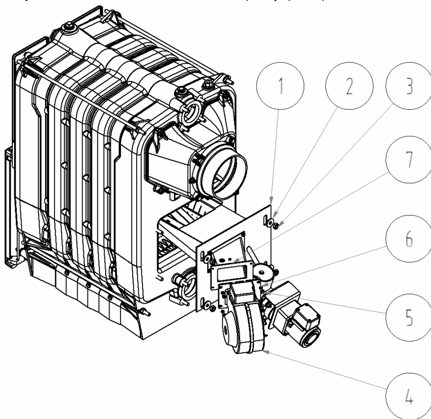
Рис. 9 Монтаж топки
