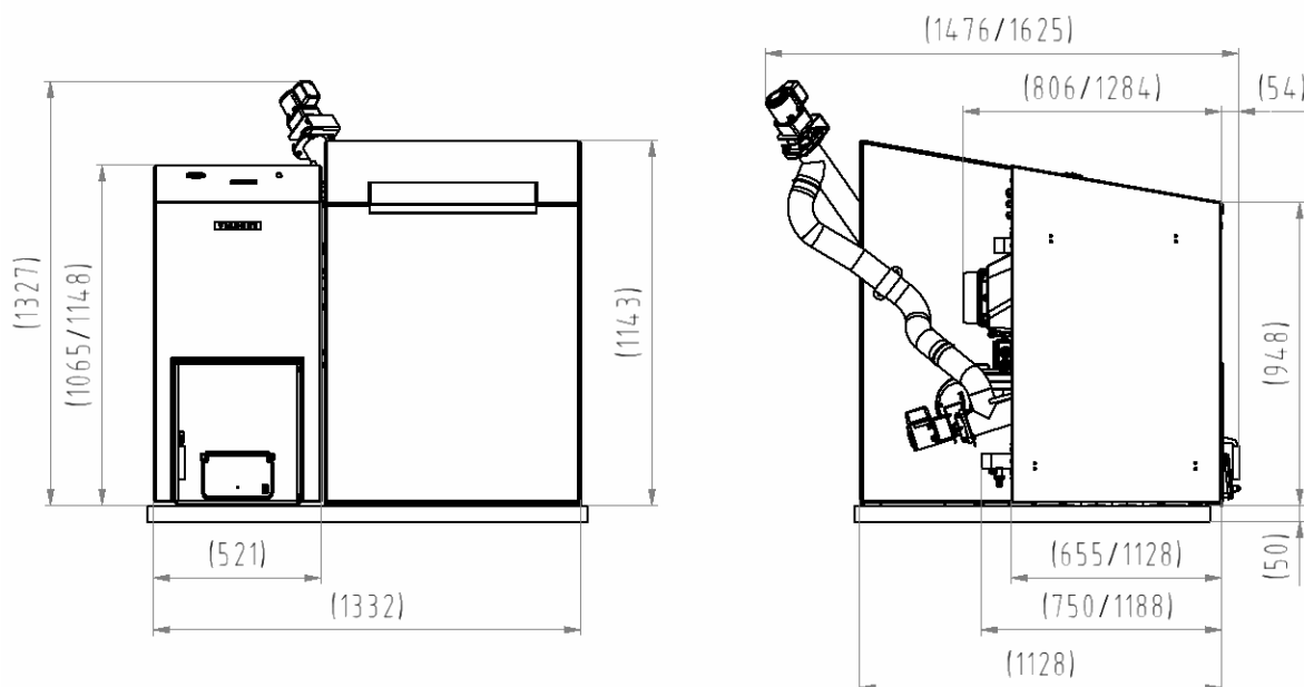
Рис. 3 Размеры котла VIADRUS HERCULES ECO (значения за дробью для версии 10 секций)
