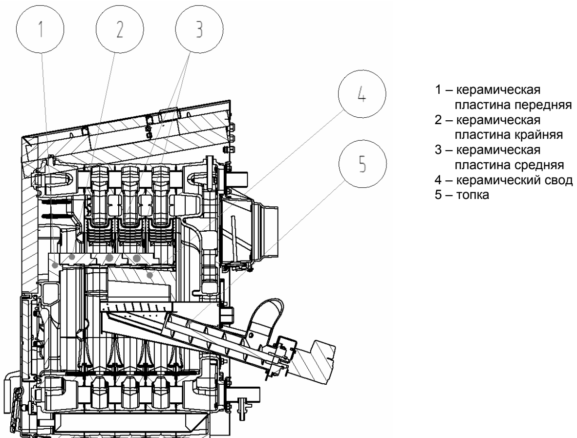
Рис. 13 Укладка керамических пластин в 5-секционный теплообменник
