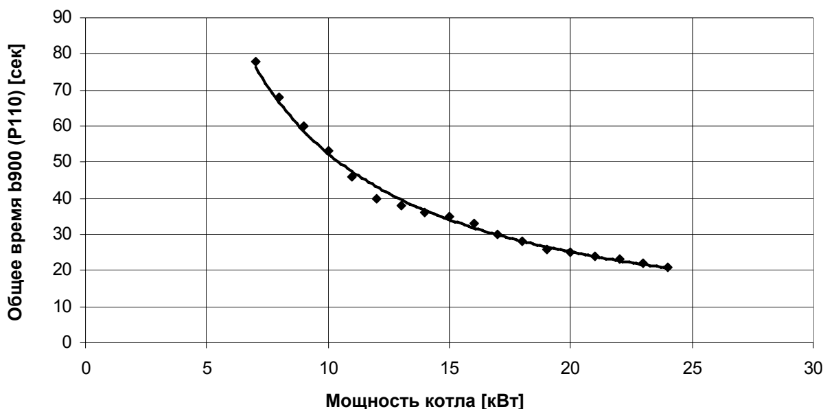
Рис. 20 График зависимости мощности котла на общем времени одного цикла при одинаковом времени подачи топлива 5 сек. Для котла VIADRUS HERCULES ECO – 5 секций.
