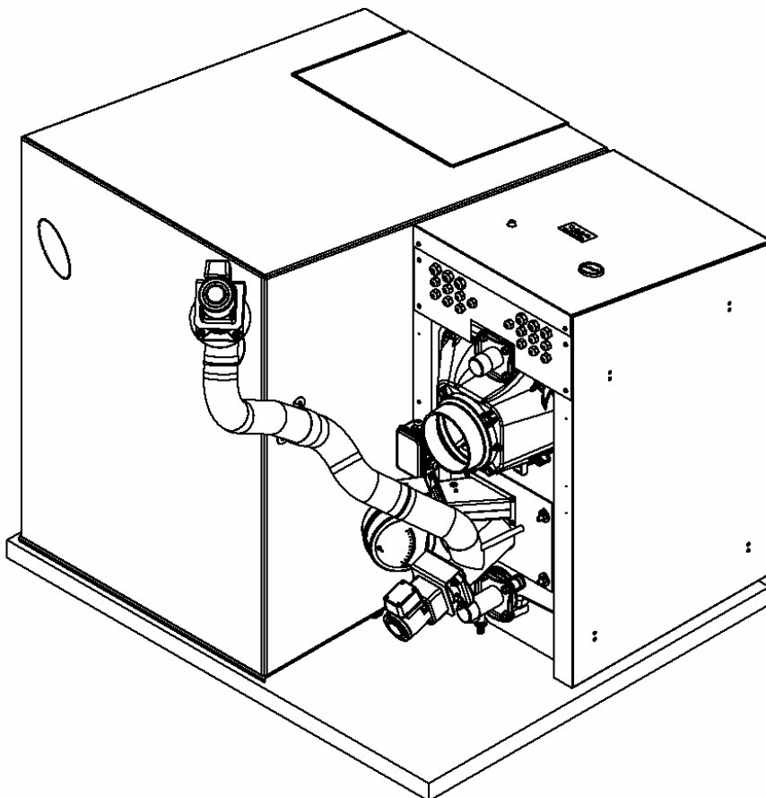
Рис. 2. Вид сзади котла VIADRUS HERCULES ECO с топливным бункером – правая версия
