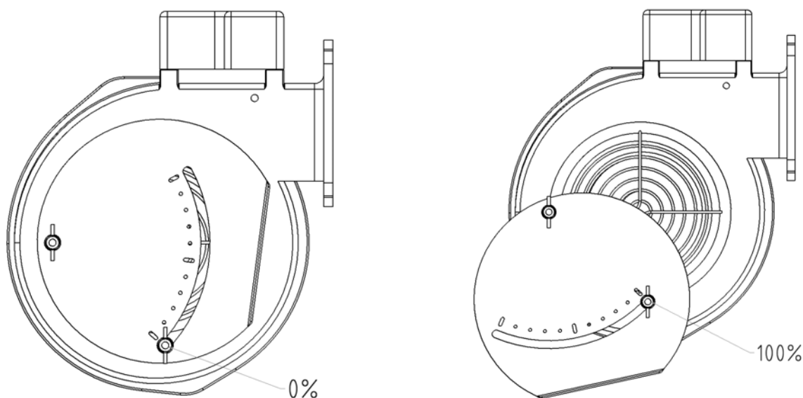
Рис. 19 Дроссельная заслонка вентилятора
