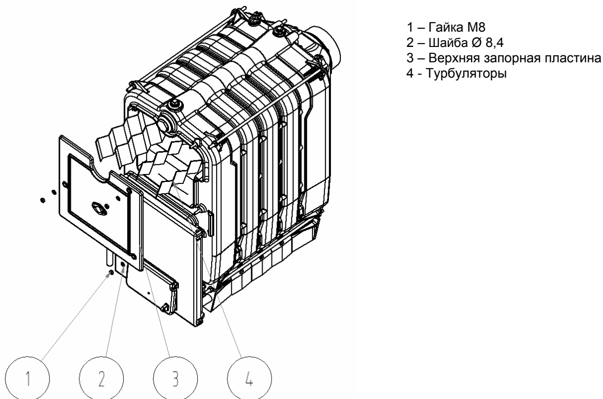
Рис. 10 Демонтаж верхней запорной пластины и установка турбуляторов
