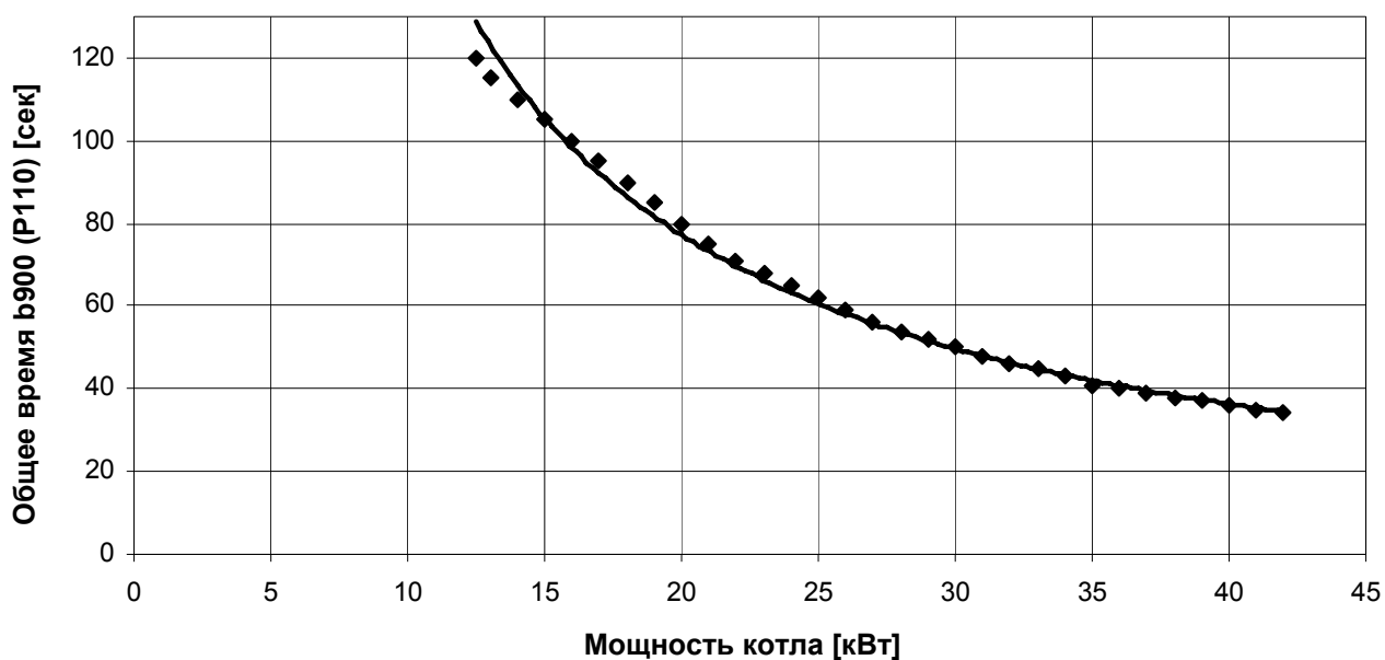
Рис. 21 График зависимости мощности котла на общем времени одного цикла при одинаковом времени подачи топлива 5 сек. Для котла VIADRUS HERCULES ECO – 10 секций.
