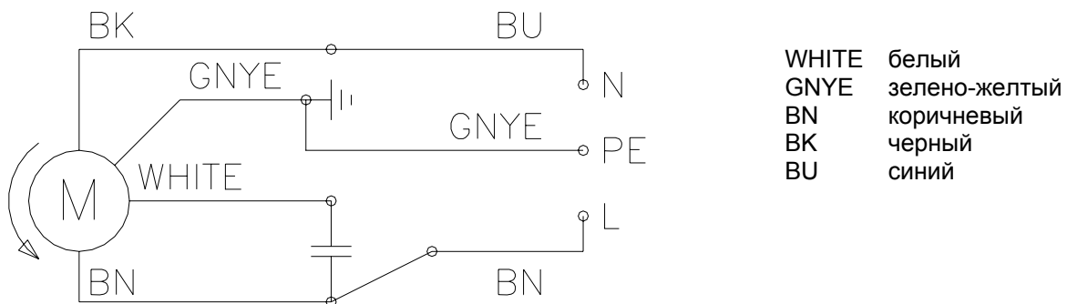
Рис. № 18 Подключение двигателей питателей
