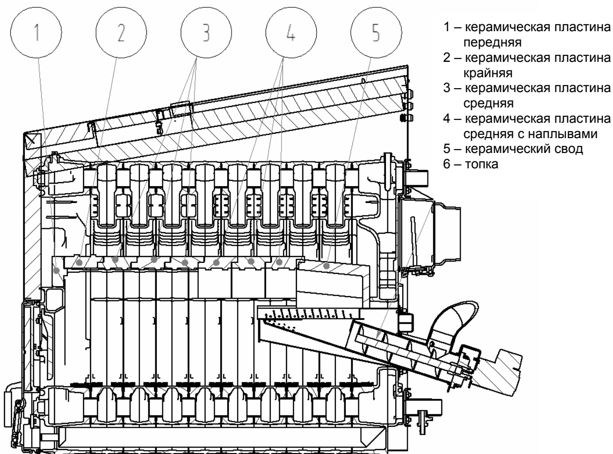
Рис. 14 Укладка керамических пластин в 10-секционный теплообменник
