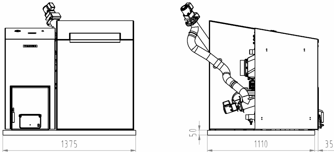
Рис. 5 Размеры цоколя под котел
