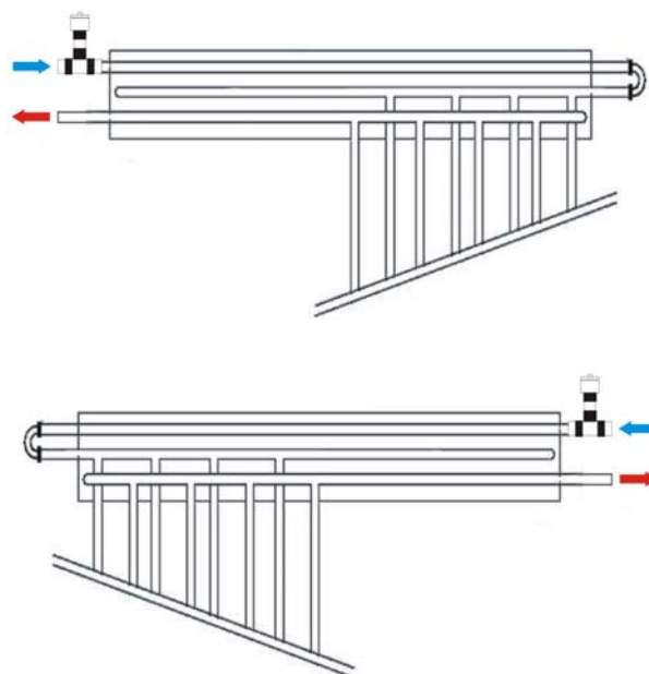
Гидравлическая схема коллекторов Space Energy
