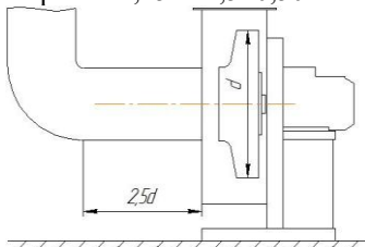
Рисунок 7 – минимальное расстояние установки всасывающего трубопровода.
