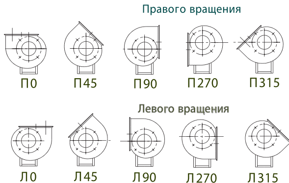
Рисунок 3 – ориентациями корпуса центробежных вентиляторов.
