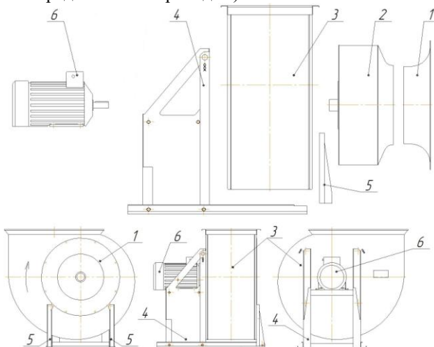
Рисунок 4 – устройство центробежных вентиляторов 1-й конструктивной схемы (с непосредственным приводом).
