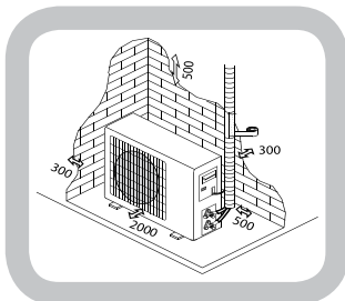
Минимальное бронирование пространство (мм) указано в рисунке
