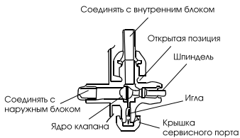
Схема четырех-ходового клапана
