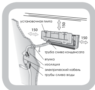
Минимальное бронирование пространство (мм) указано в рисунке
