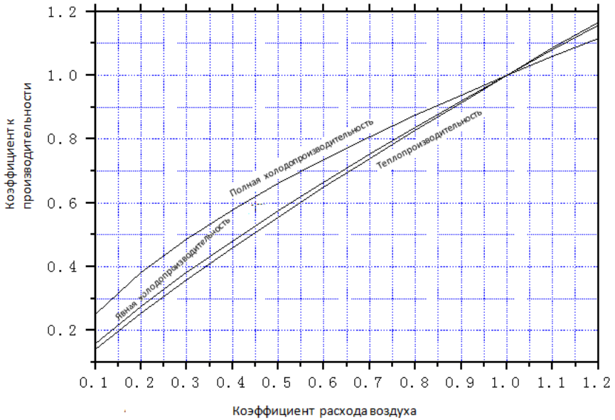
График пересчета коэффициента холодопроизводительности
