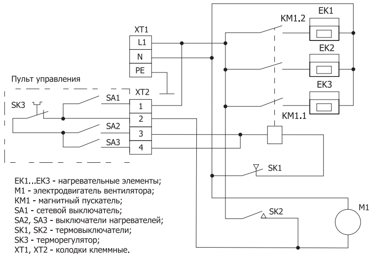
Рис. 2. Схема электрическая ST 508
