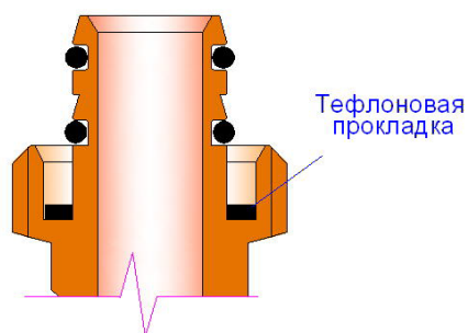
Рис.3.3.4.р.1 Диэлектрическая прокладка на штуцере фитинга
