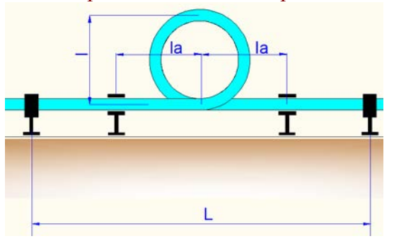
Петлеобразный компенсатор
