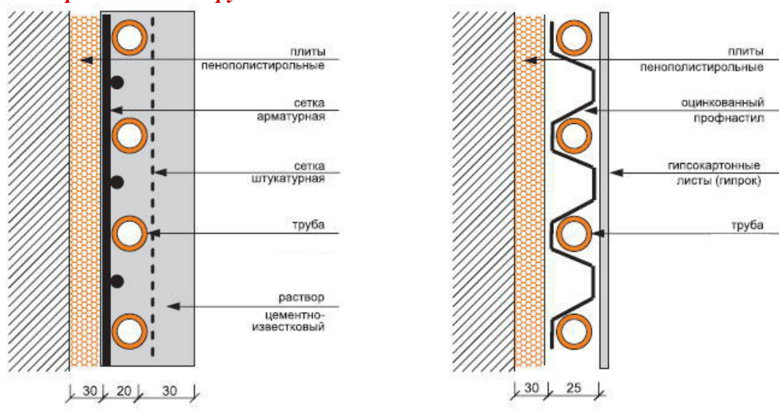
Рис.5.4.р.6 Варианты конструктивного исполнения теплых стен
