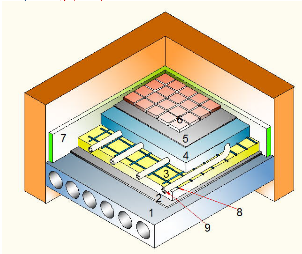
Рис. 5.3.1.3. п.1 Конструкция «мокрого» теплого пола
