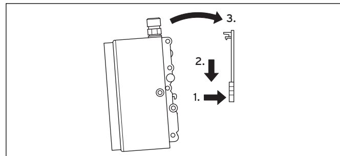
Obr. 3.4 Pripevnenie zariadenia
