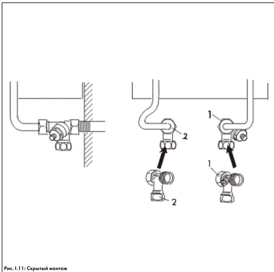
Рис. 1.11: Скрытый монтаж
