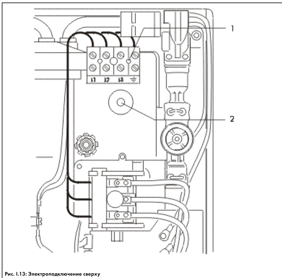
Рис. 1.13: Электроподключение сверху
