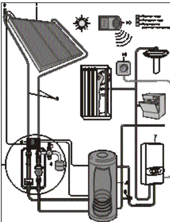
Рис.А.1 Функциональная схема VED.../5 E exclusiv LCD
