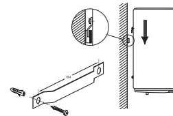
(Рис. 2) Установка
