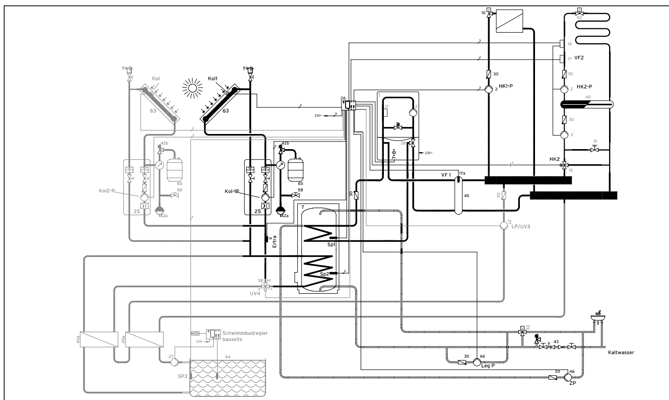
Рис. 4.10 Гидравлическая схема 3.2
