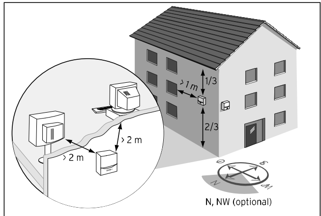
Рис. 3.5: Место установки приемника DCF
