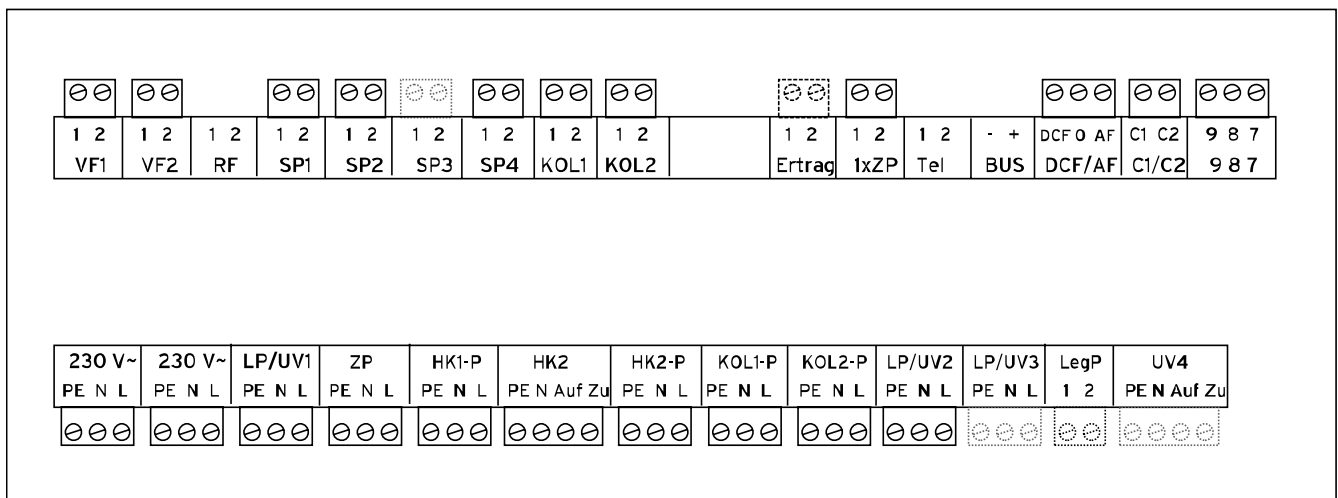
Рис. 4.25 Используемые гнезда системы штекерных разъемов ProE
