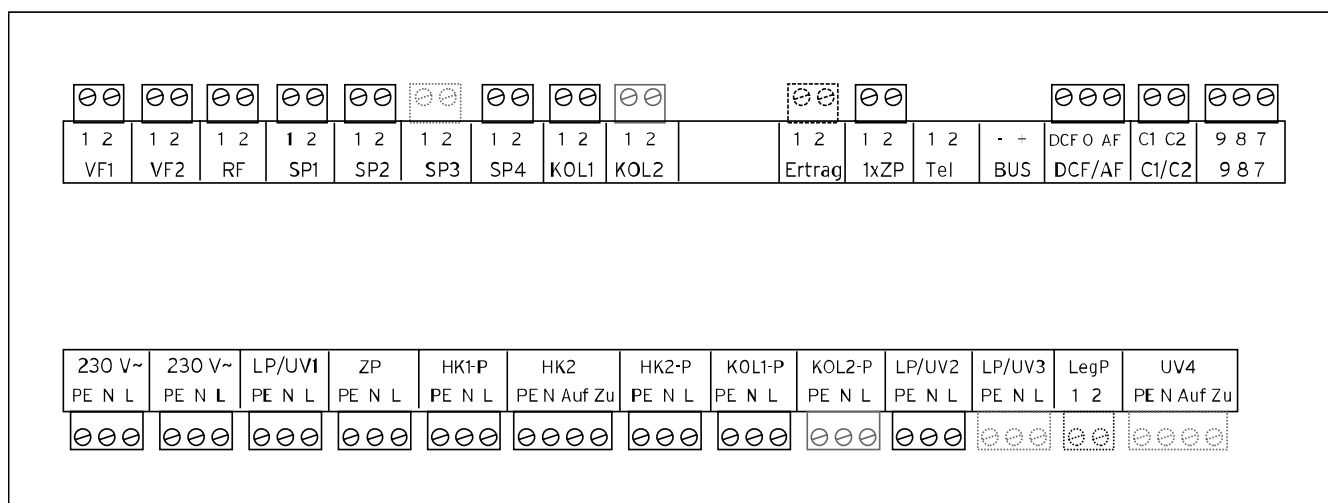
Рис 4.11 Используемые гнезда системы штекерных разъемов ProE
