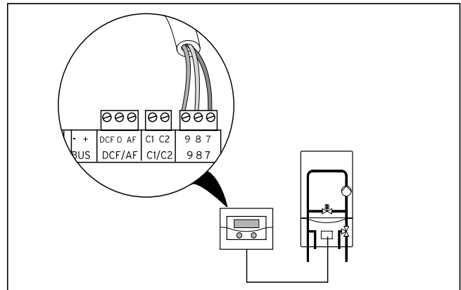
Рис. 4.1 Подключение нагревательного прибора
