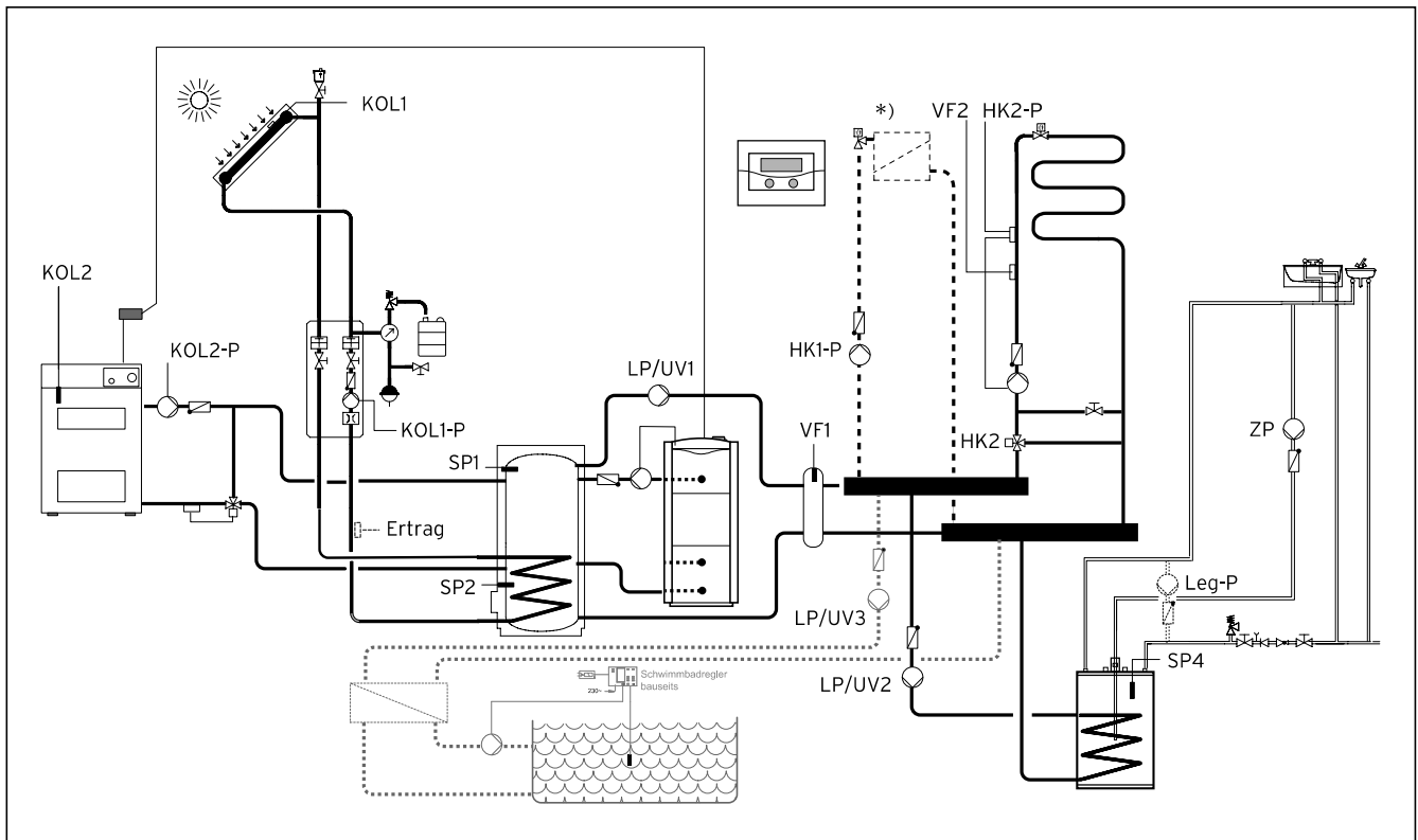
Рис. 4.24 Гидравлическая схема 8
