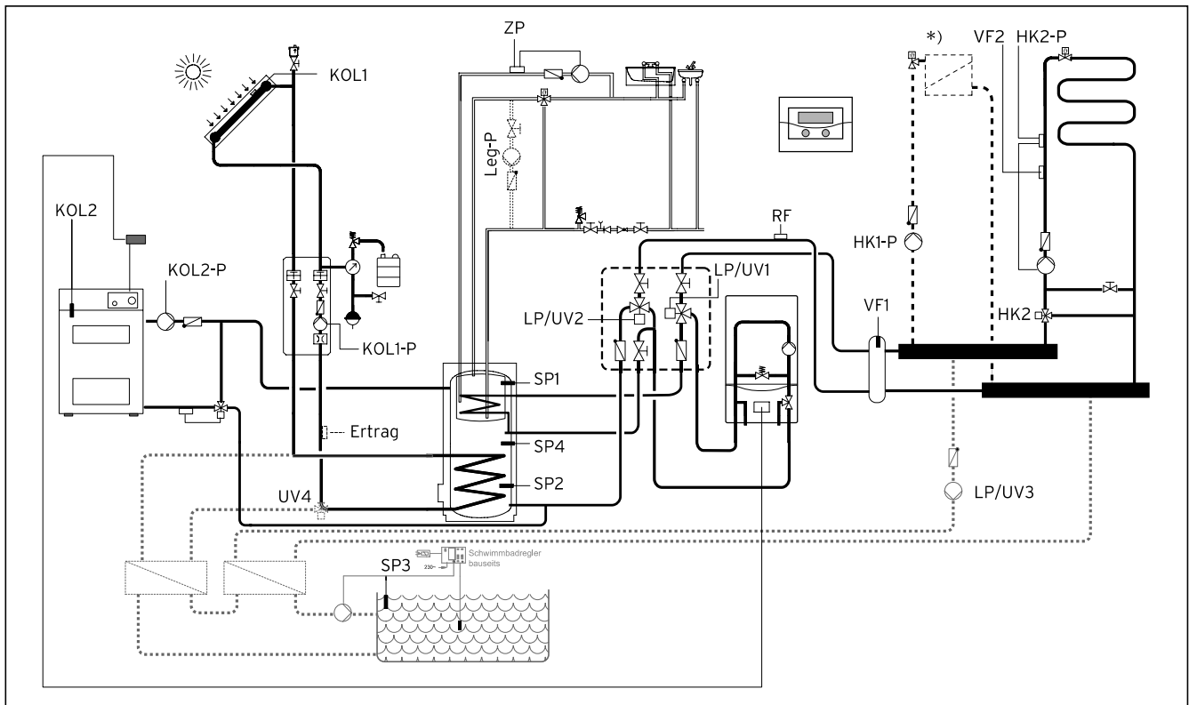
Рис. 4.4 Гидравлическая схема 2
