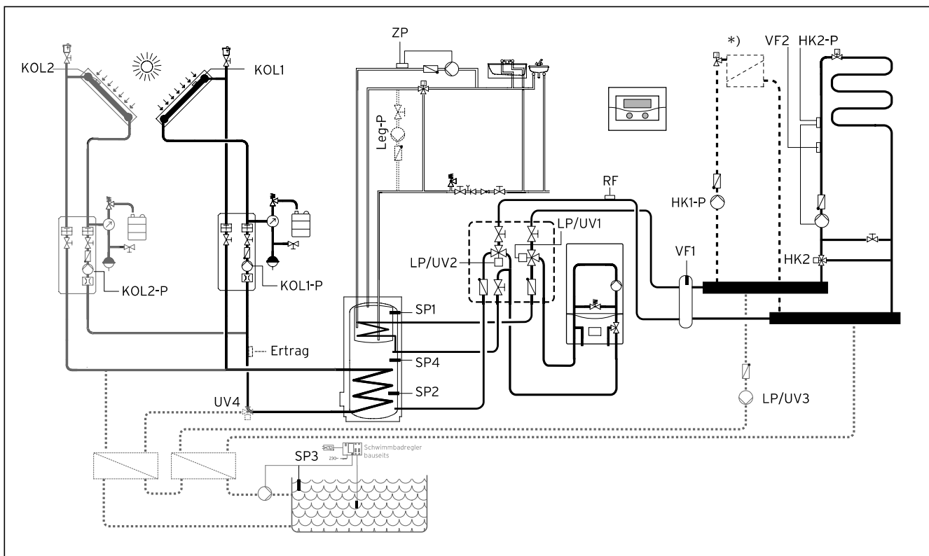
Рис. 4.2 Гидравлическая схема 1
