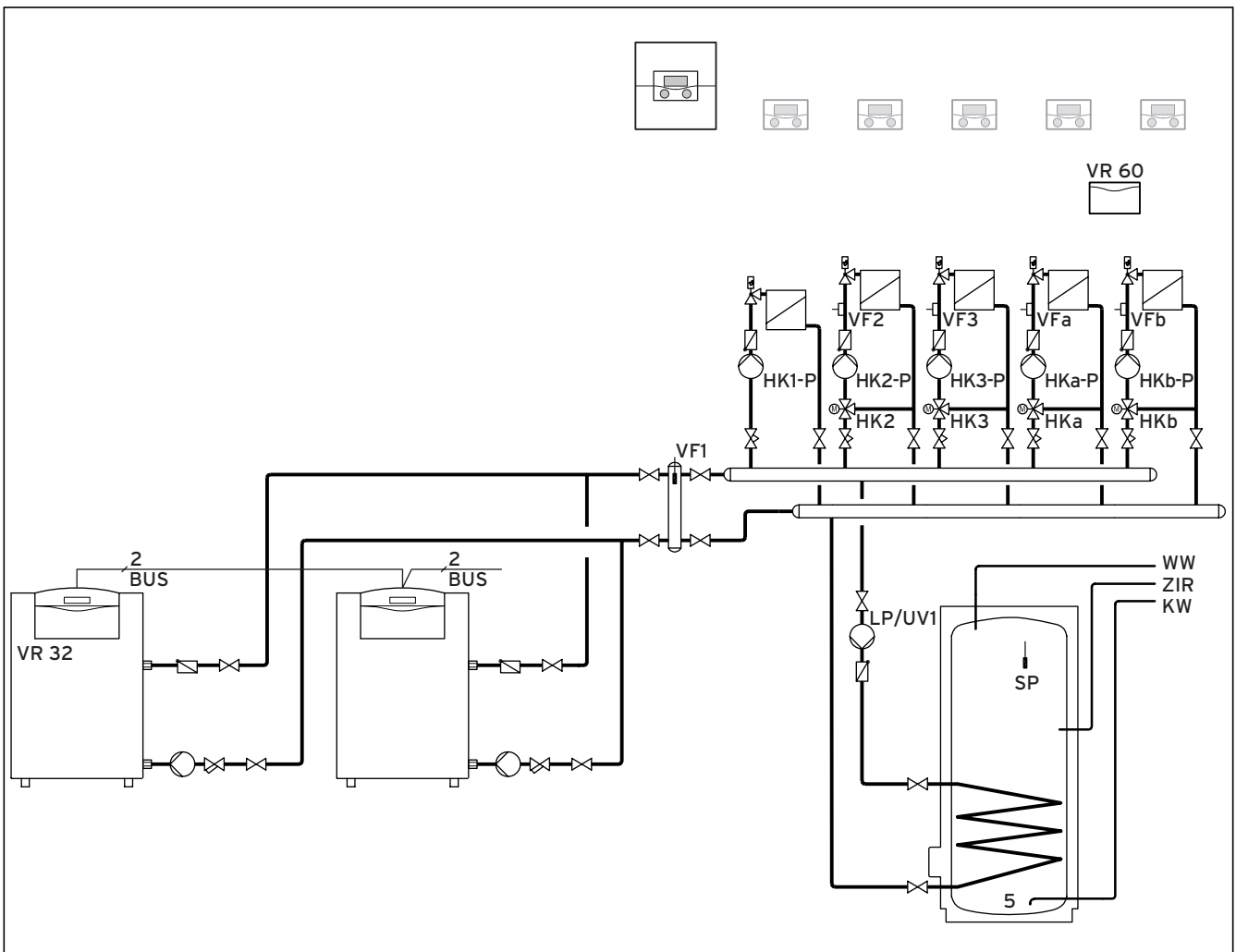
Рис. 5.10 calorMATIC 630 в комбинации с двумя котлами ecoCRAFT
